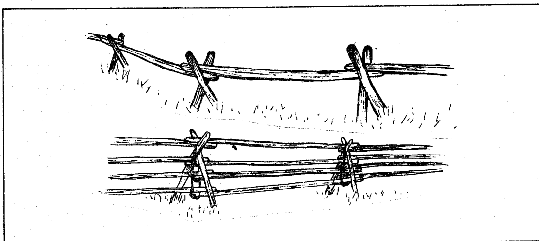
Clôtures à chevalets.
